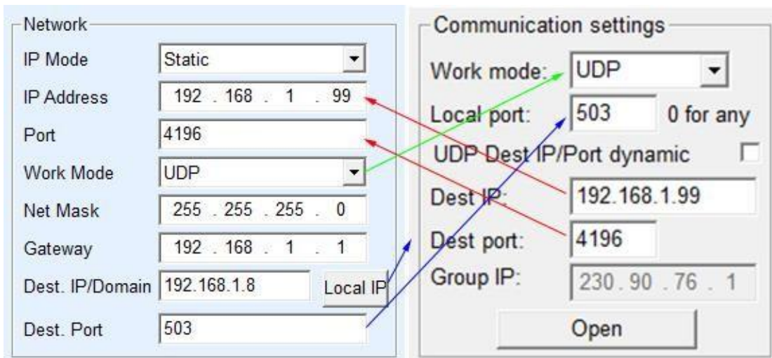
Figure 18 UDP mode parameter configuration
