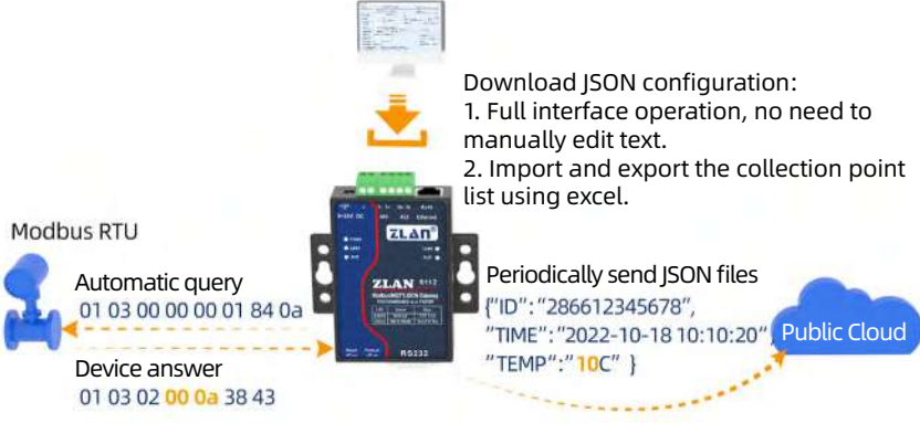
JSON configuration
